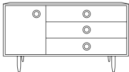
halo m1
