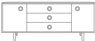
halo m2
